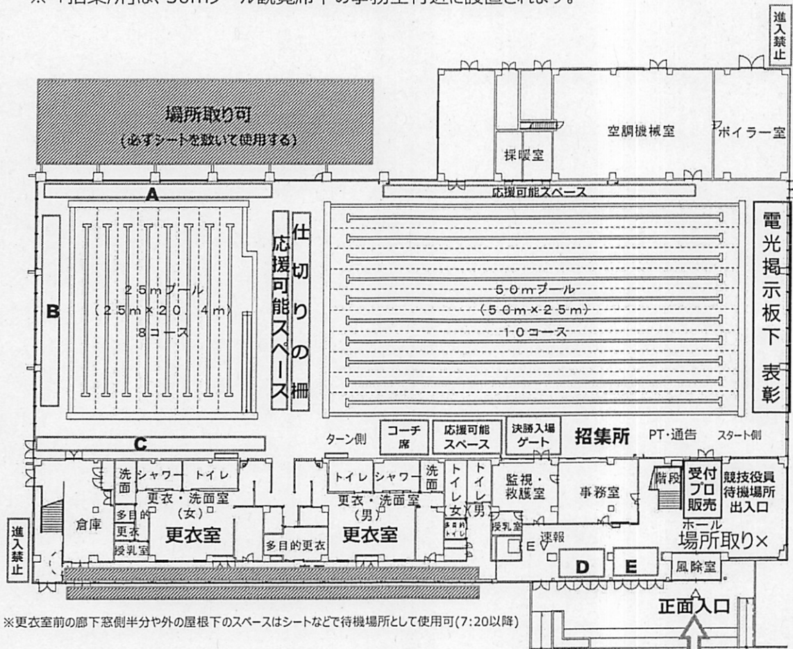
1階平面図 選手、保護者入口
